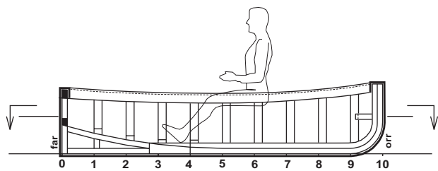
fenékszerkezet
