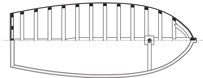
fedélzeti szerkezet
