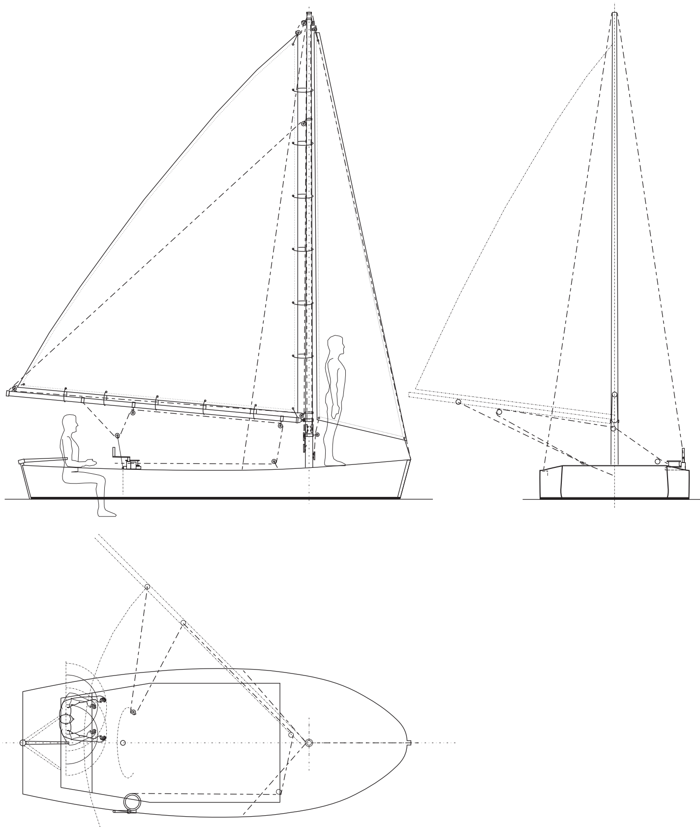
BBBZ5 vitorlás csónak M1:50 3. lap: Vitorlák és kötelek
